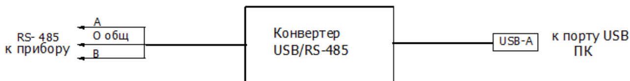
Рисунок 2 - Схема подключения конвертера USB/RS-485G
